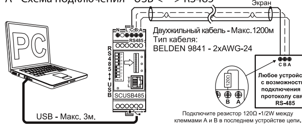
А - Схема подключения - USB <--> RS485
